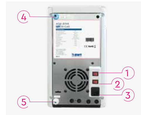
Fig. 3: Parte trasera de AQA drink Pro 20 CAS
