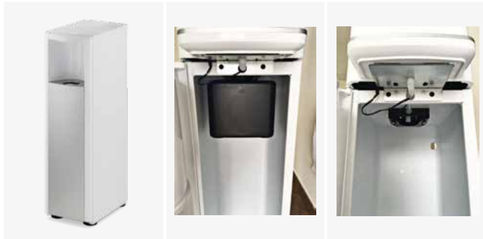
Fig. 4 : socle de l'AQA drink Pro 20 (vue de l'extérieur)
