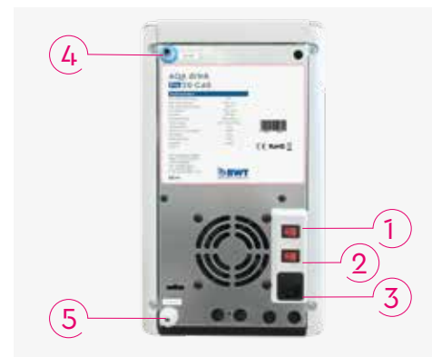
Fig. 3: Parte traseira do AQA drink Pro 20 CAS
