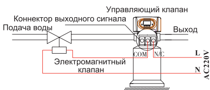
Рис. 3-2 Цепь управления электромагнитным клапаном на входе
