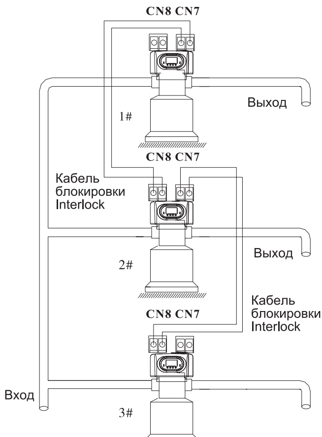
Рисунок 3-10. Одновременная подача воды и поочередная регенерация
