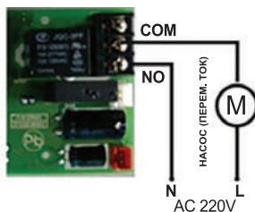
Рисунок 3-7. Электрическое подключение подкачивающего насоса на входе напрямую
