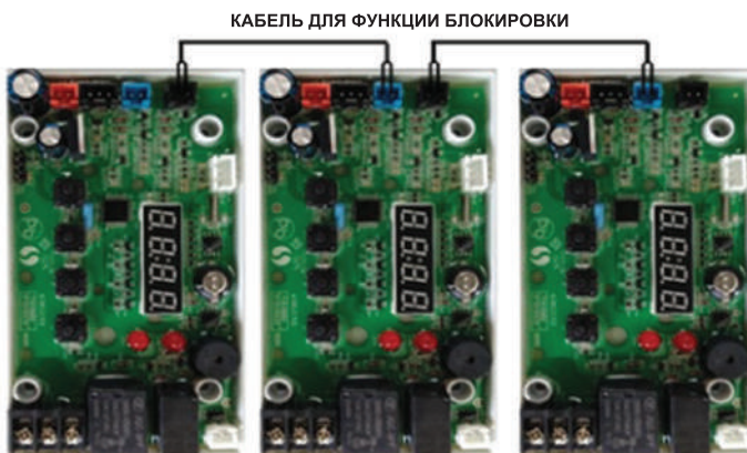
Рисунок 3-9. Электрическое подключение для функции блокировки
