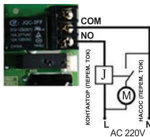
Рисунок 3-8. Электрическое подключение подкачивающего насоса на входе через контактор
