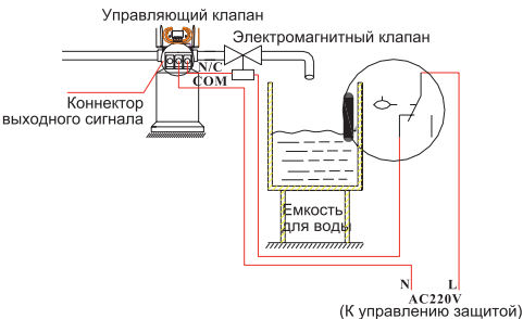
Рисунок 3-1 Электрическое подключение электромагнитного клапана на выпускном трубопроводе
